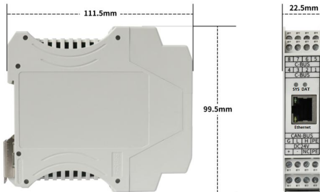
图 2.1 GCAN-205C 模块外形尺寸
