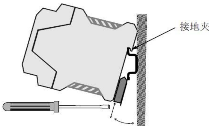
图 2.2 GCAN-205C 模块安装
