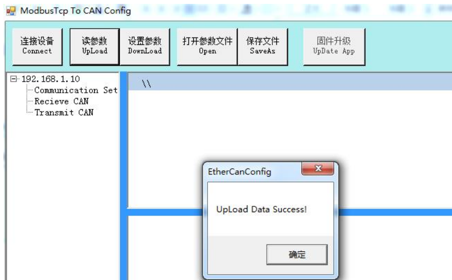
图 4.4 配置软件读参数成功
