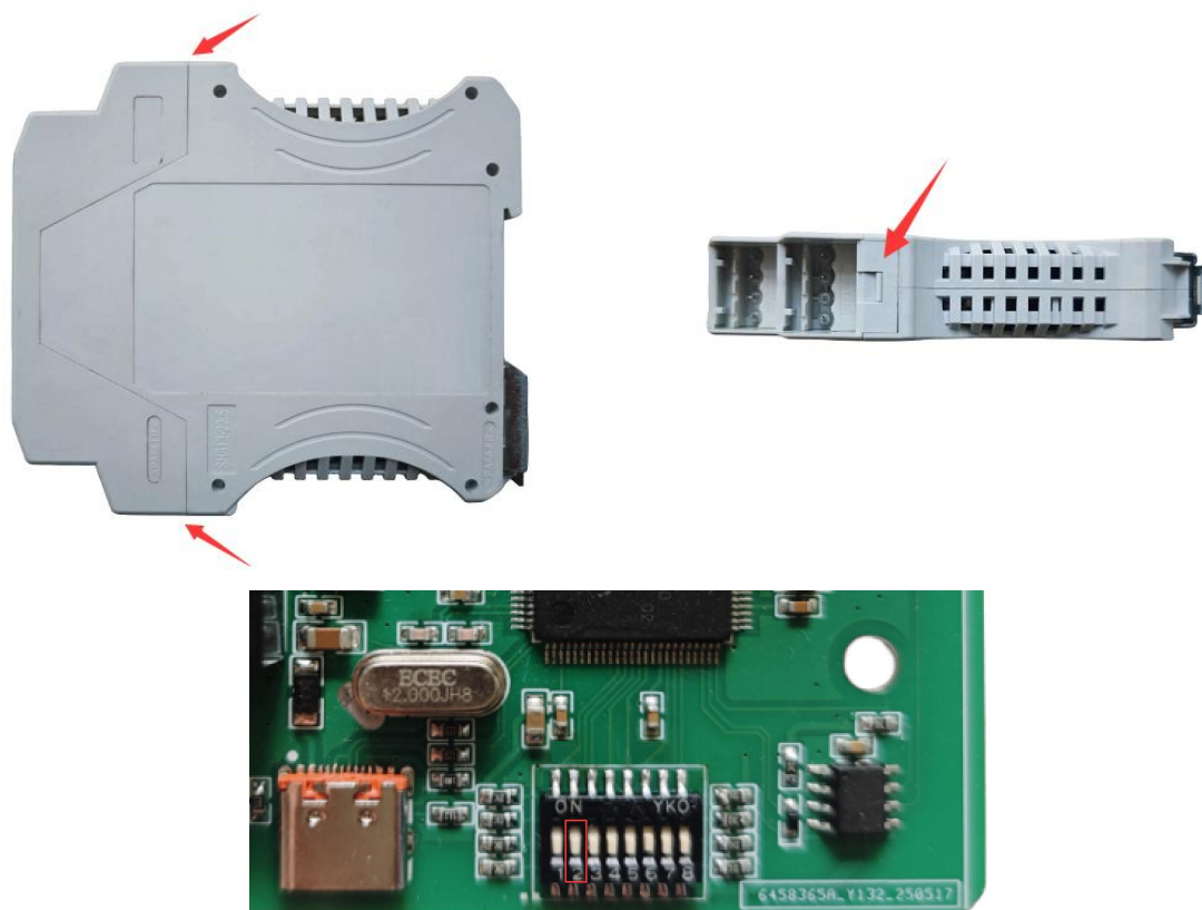
图4.1 GCAN-205C恢复出厂设置
