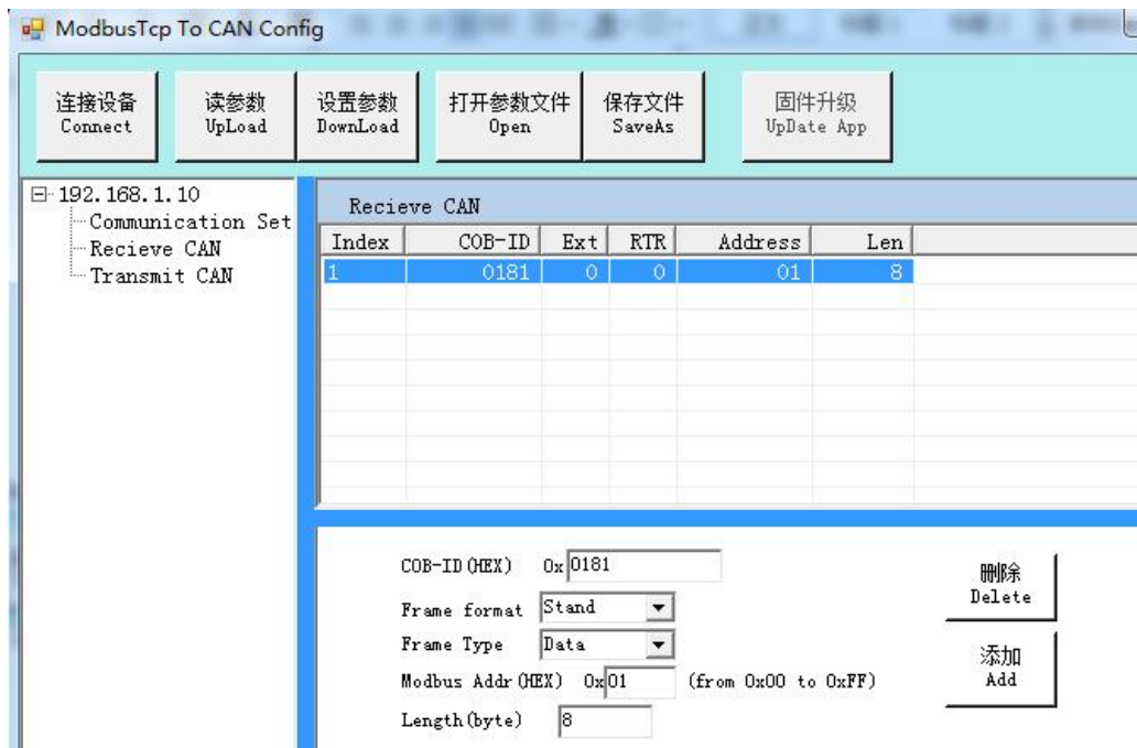
图 4.5 “Receive CAN”设置界面
