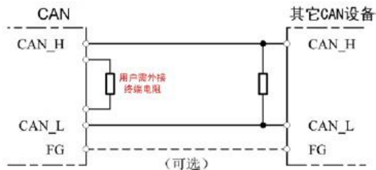
图3.5 GCAN-205C模块与其他CAN节点设备连接
