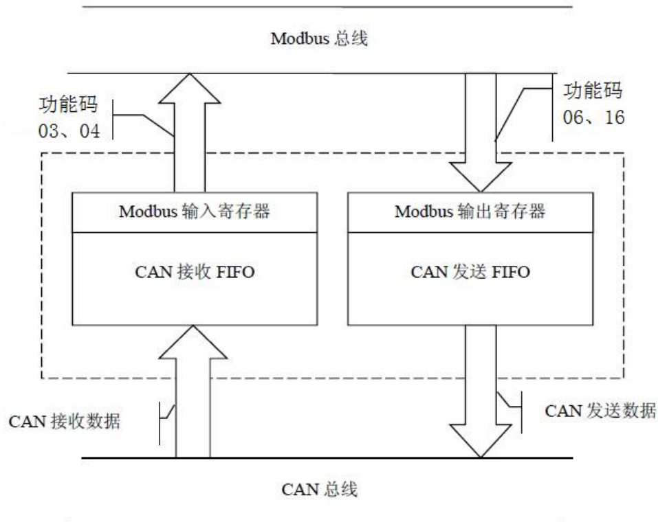
图 3.1 GCAN-205C 模块工作原理
