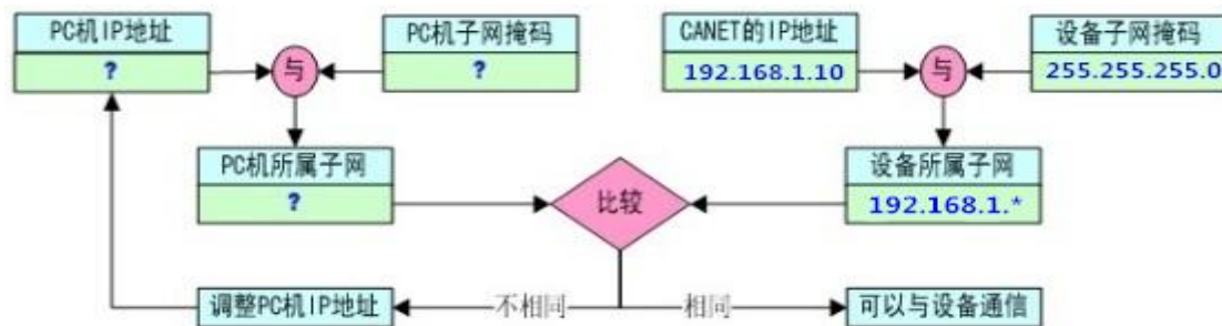
图 3.2 PC 机与 GCAN-205C 模块是否处于同一网段检测流程
