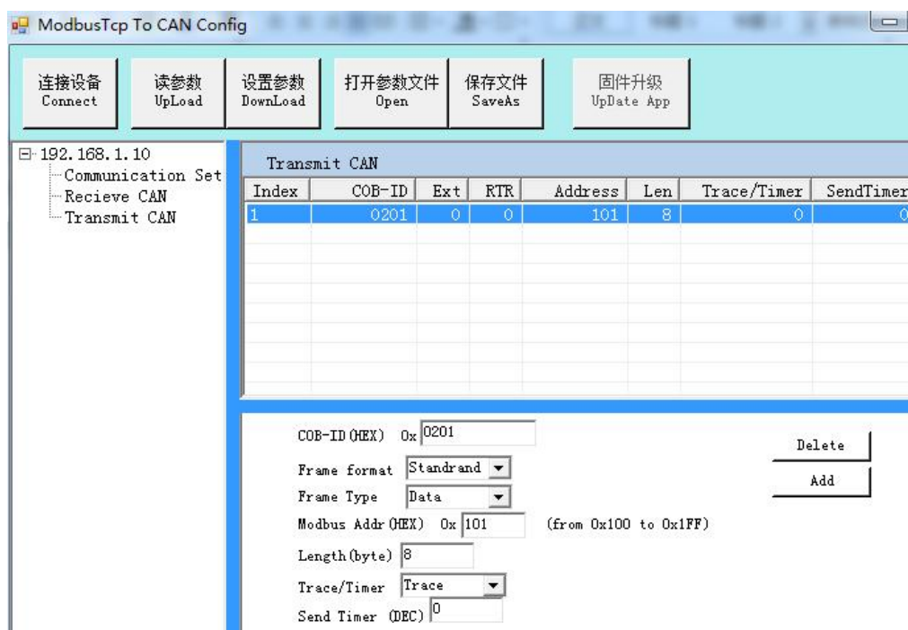
图 4.6 “Transmit CAN” 配置界面
