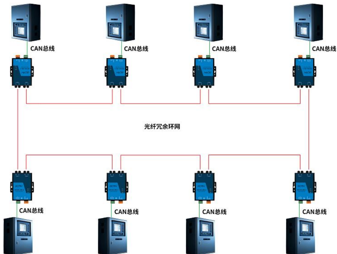
GCAN-208-2C 典型应用——环网
