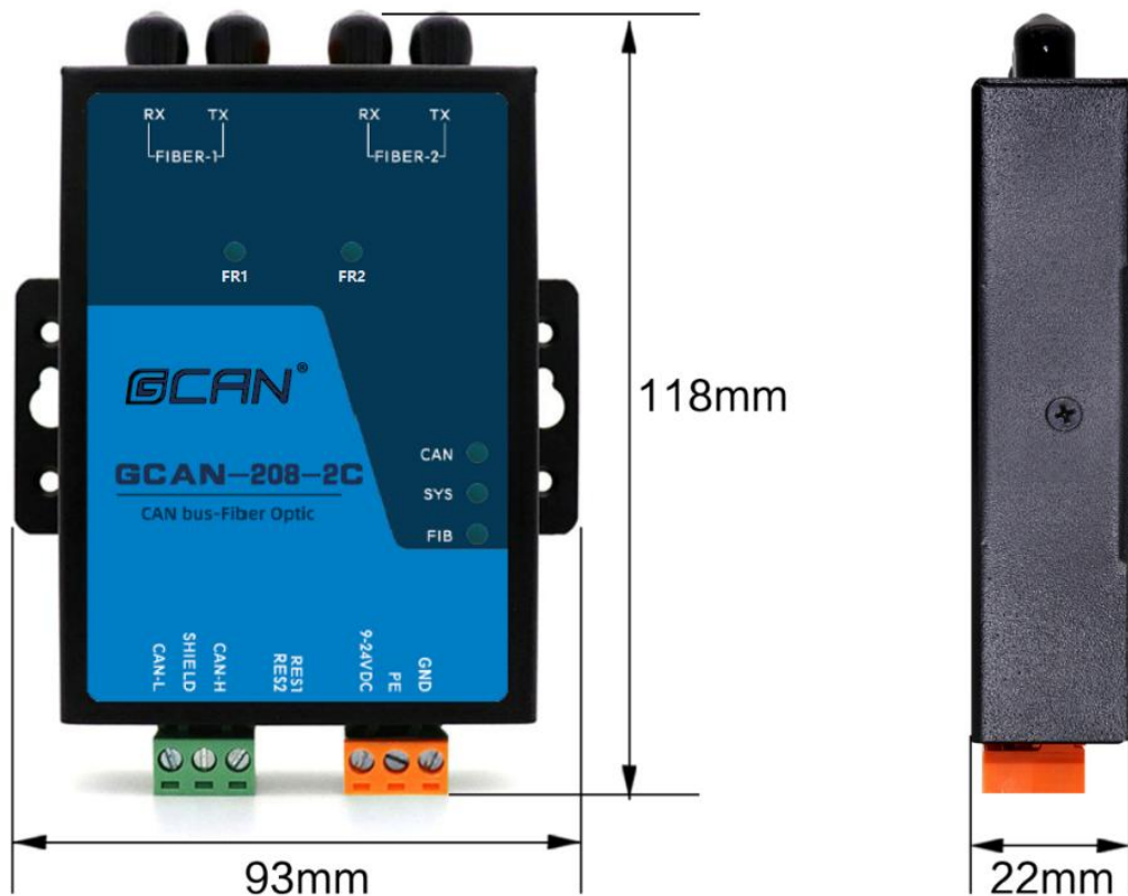
图 2.1 GCAN-208-2C 外形尺寸
