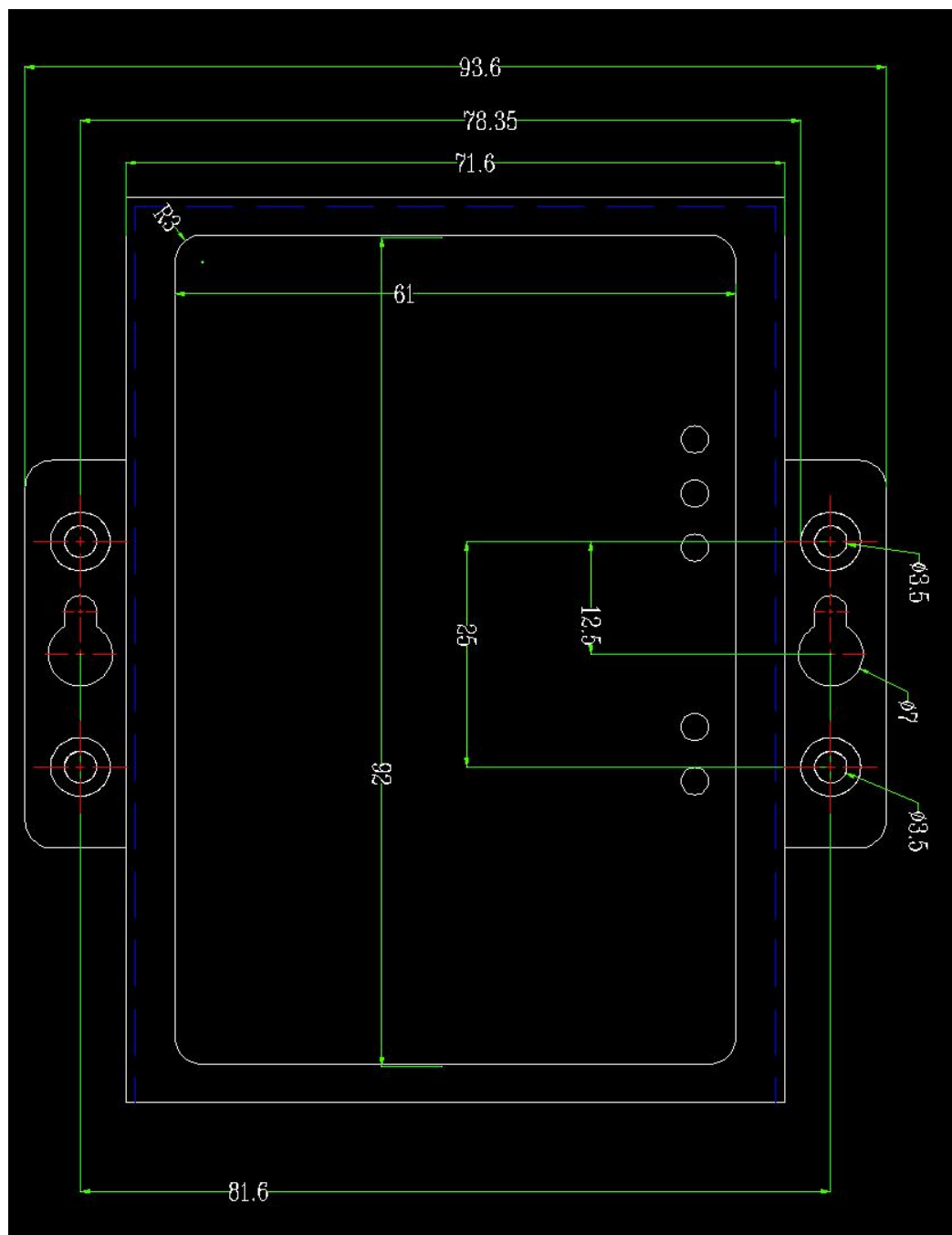
图 2.2 GCAN-208-2C 系列模块机械尺寸示意图
