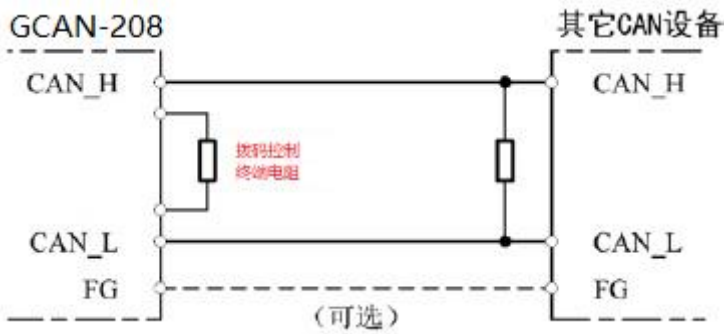
图 3.8 GSCAN-208-2C 系列模块与其他 CAN 节点设备连接
