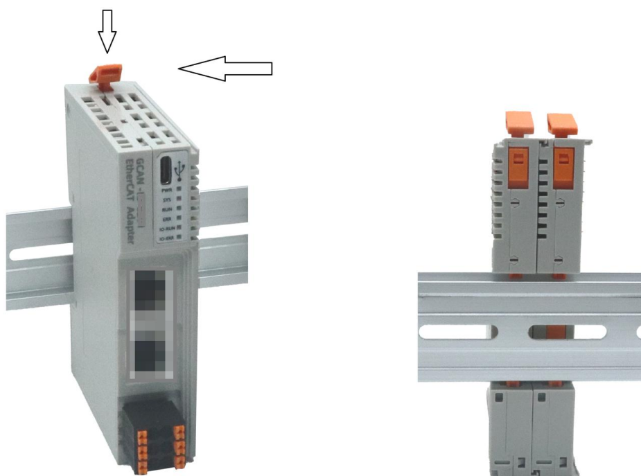
图 2.3 GCAN-PLC-325 可编程逻辑控制器模块安装
