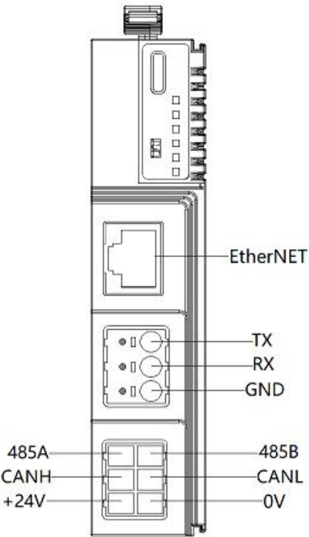
图 2.7 GCAN-PLC-325 总线及电源接线端子排
