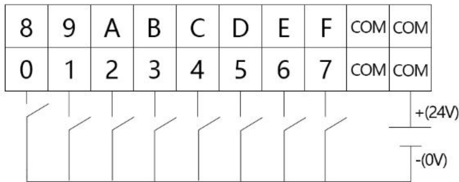
图 2.6 GCAN-PLC-200 DI（0-7 路）漏型接线
