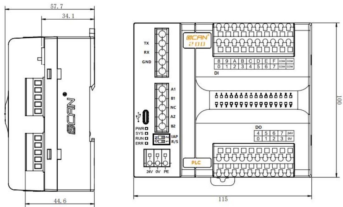
图 2.1 GCAN-PLC-200 模块外形尺寸图
