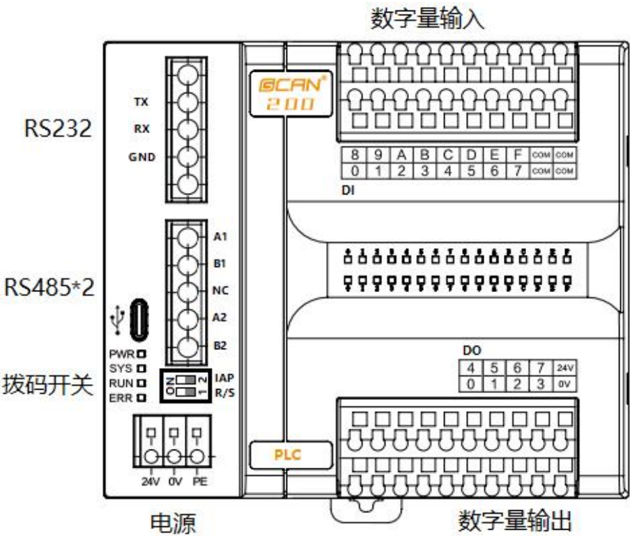
图 2.4 GCAN-PLC-200 各接口位置
