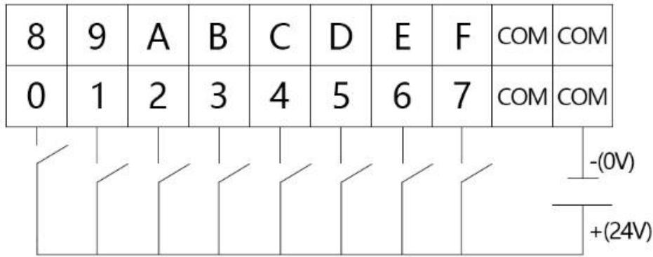
图2.7 GCAN-PLC-200 DI（0-7路）源型接线
