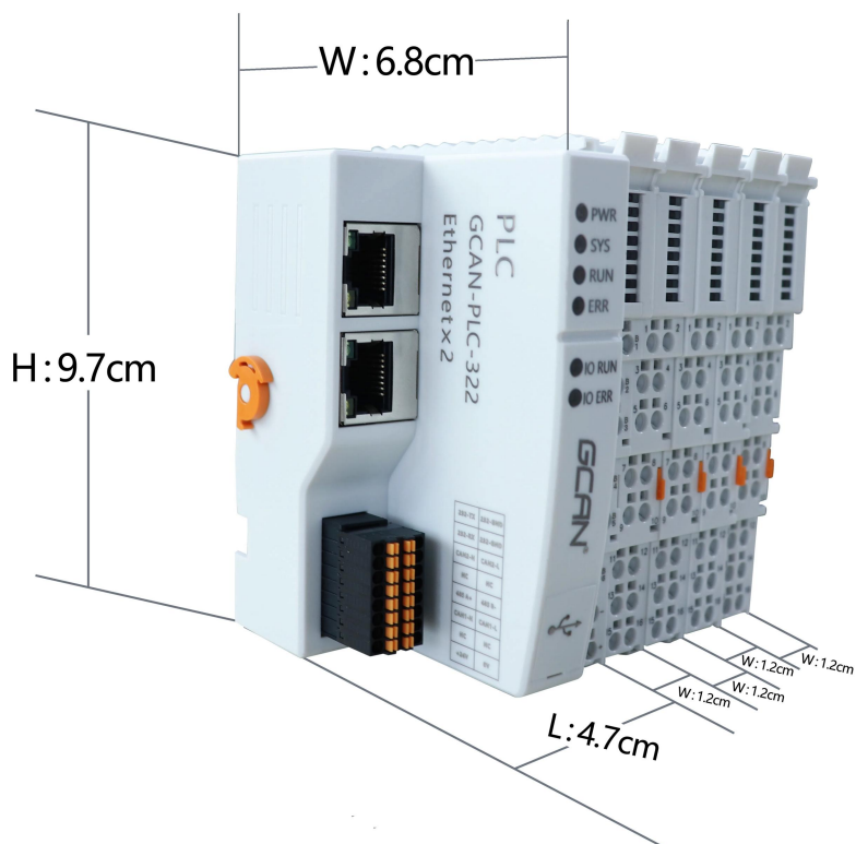
图 2.2 GCAN-PLC-322 外观尺寸图
