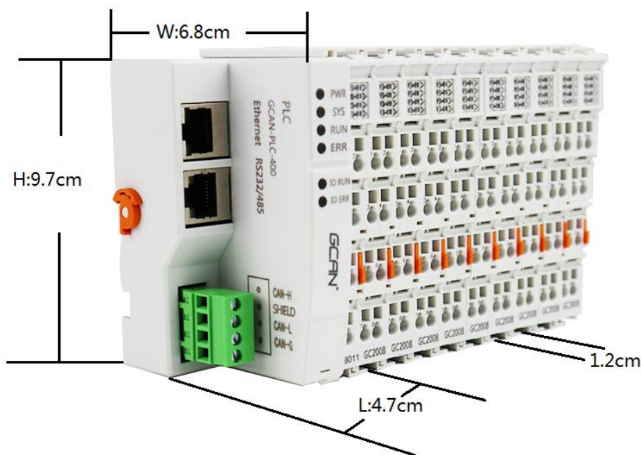
图 2.1 GCAN-PLC-400 外观尺寸图
