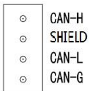
图 2.7 GCAN-PLC-400 的 CAN 总线端子排
