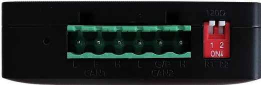
图 2.3 CAN-bus 接口位置
