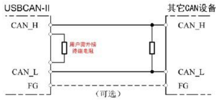
图 3.2 USBCAN-II Pro+与其他 CAN 节点设备连接
