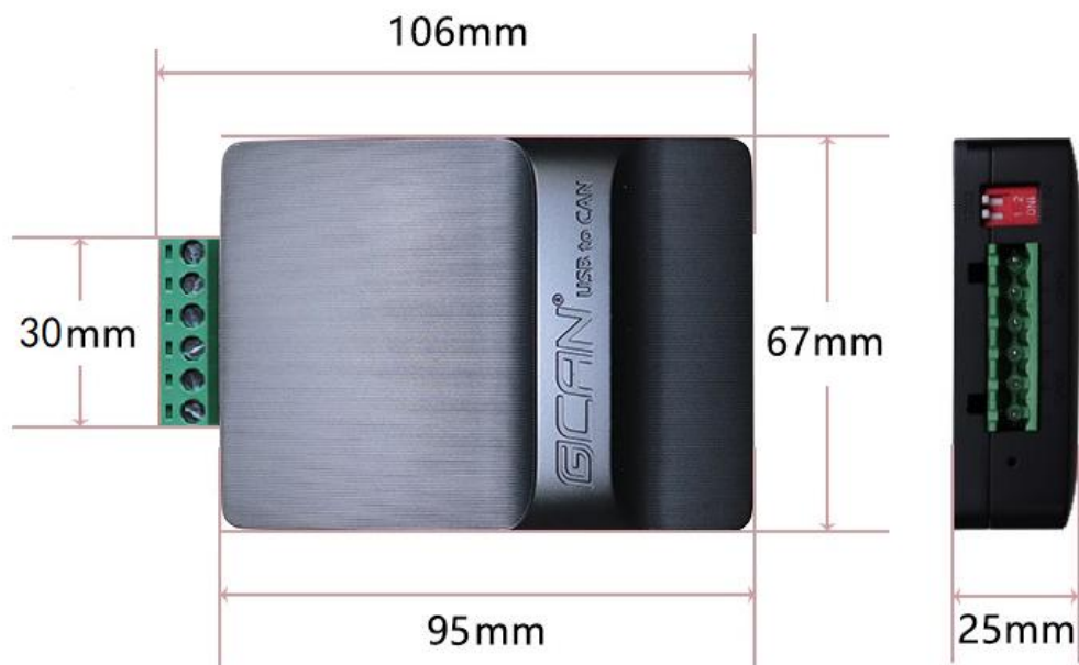
图 2.1 USBCAN-II Pro+外形尺寸
