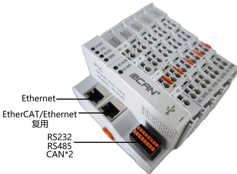
图 2.6 GCAN-PLC-522 的总线接口样式
