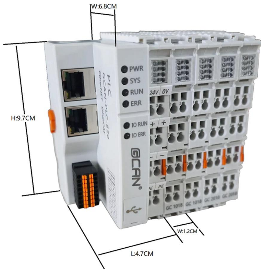
图 2.1 GCAN-PLC 外观及尺寸图
