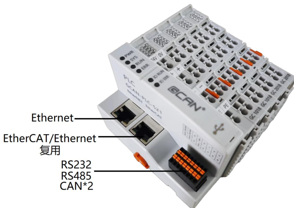
图 2.6 GCAN-PLC-521 的总线接口样式
