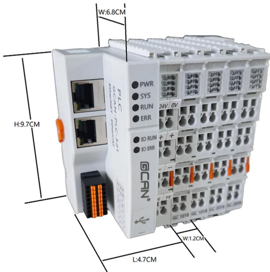
图 2.1 GCAN-PLC 外观及尺寸图
