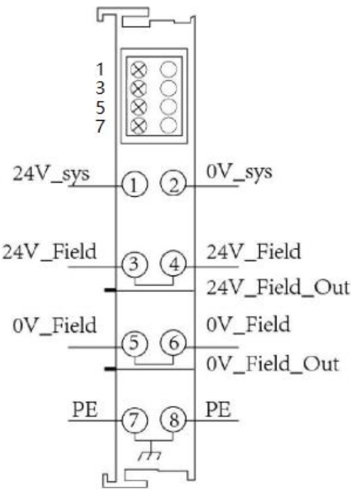
图 2.8 PLC 主控模块电源接线端子排
