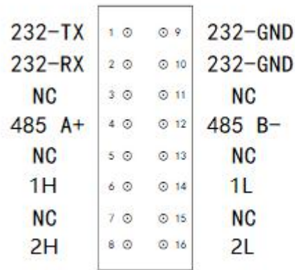
图 2.7 GCAN-PLC-521 的总线接口样式
