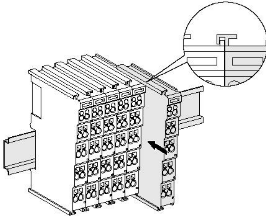
图 2.2 GCAN-PLC 安装
