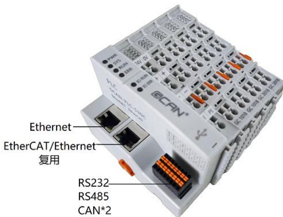
图 2.6 GCAN-PLC-530C 的总线接口样式
