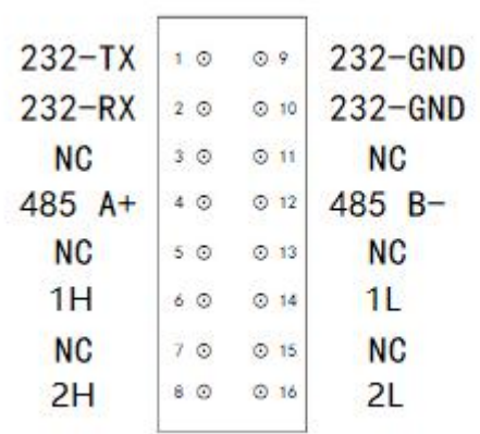
图 2.7 GCAN-PLC-530C 的总线接口样式
