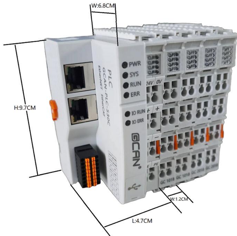
图 2.1 GCAN-PLC 外观及尺寸图
