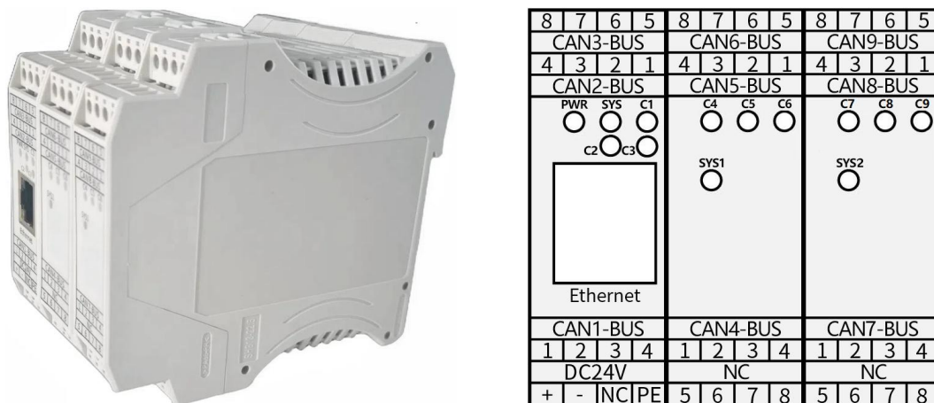
图 2.5 GCAN-GT-418-9 系列模块接线端子排
