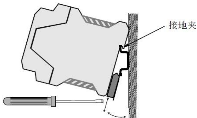
图 2.2 GCAN-GT-418 系列模块安装
