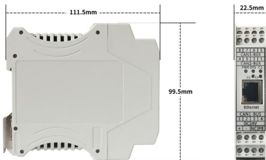
图 2.1 GCAN-GT-418-3/3R/3C 模块尺寸图
