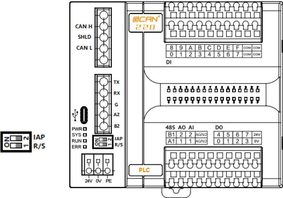
4.1 GCAN-PLC-220 拨码开关图
