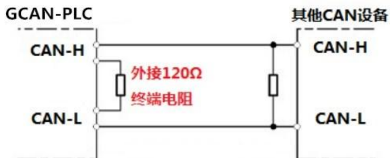
图 3.3 GCAN-PLC-220 与其他 CAN 节点设备连接
