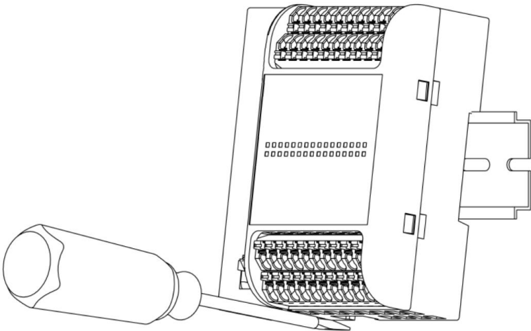
图 2.3 GCAN-PLC-220 CANopen 模块拆卸
