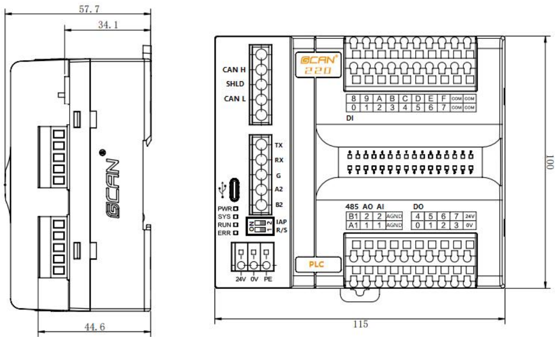
图 2.1 GCAN-PLC-220 模块外形尺寸图
