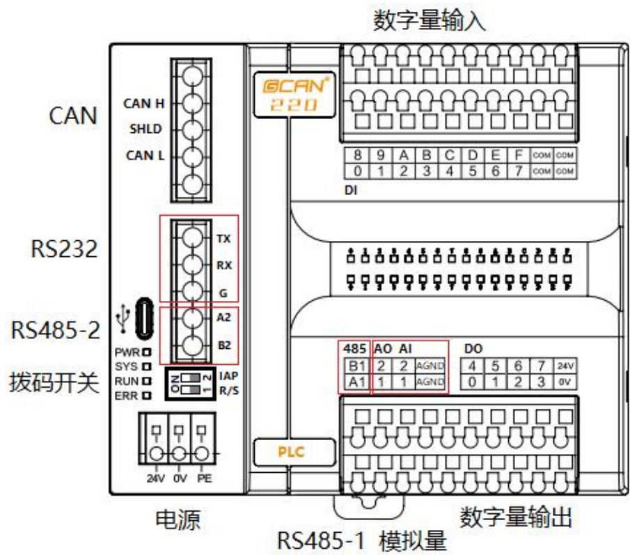
图 2.4 PLC-220 各接口位置
