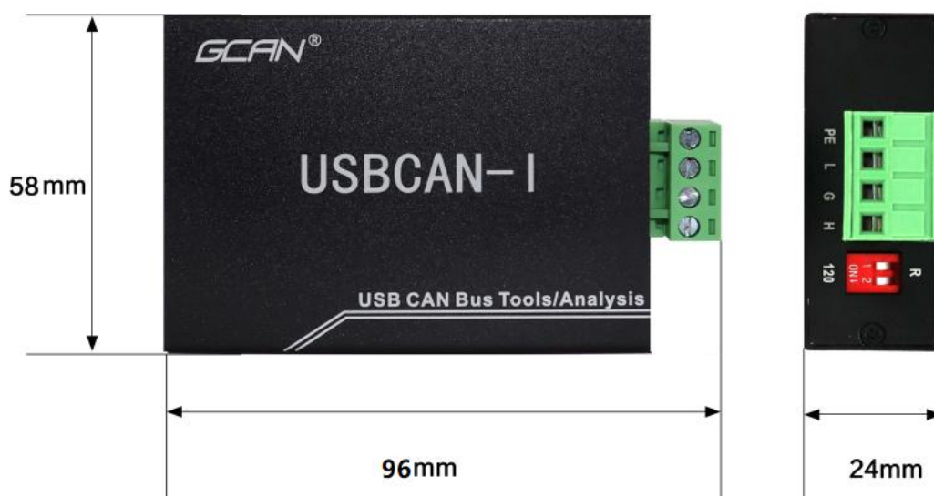
图 2.1 USBCAN-I Pro 外形尺寸
