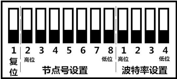
图 2.4 GCAN-4057 模块拨码开关
