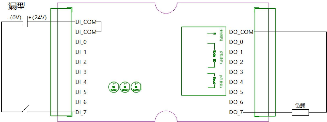
图 2.5 GCAN-4057 模块漏型输入、PNP 输出接线图
