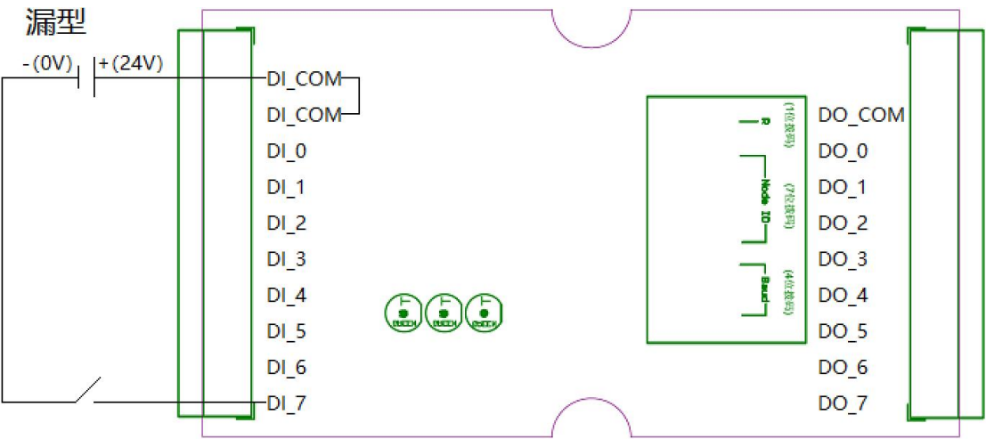
图 C.2 漏型数字量输入接线示意图
