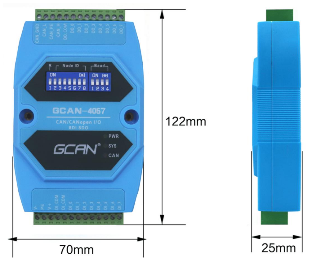
图 2.1 GCAN-4057 外形尺寸
