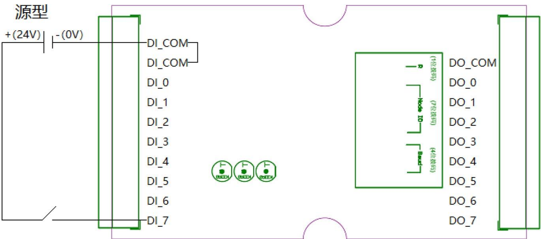
图 C.1 源型数字量输入接线示意图
