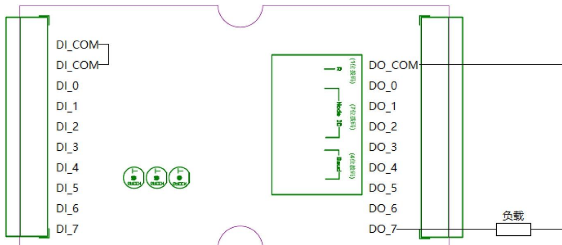
图 C.3 数字量输出接线示意图
