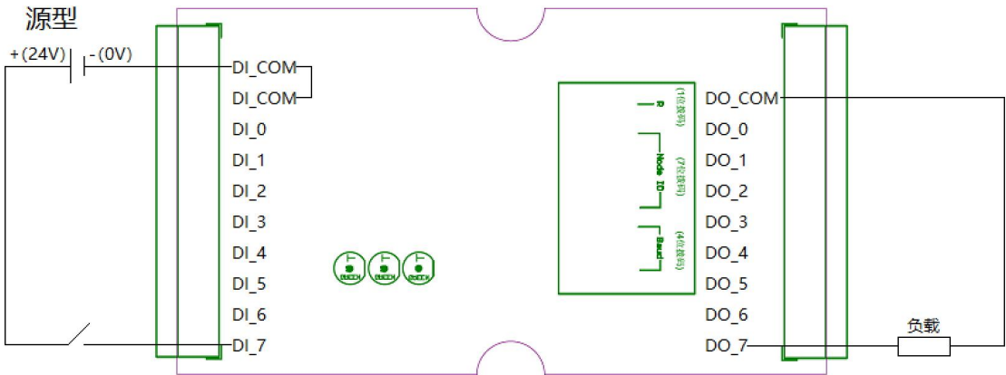
图 2.4 GCAN-4057 模块源型输入、PNP 输出接线图
