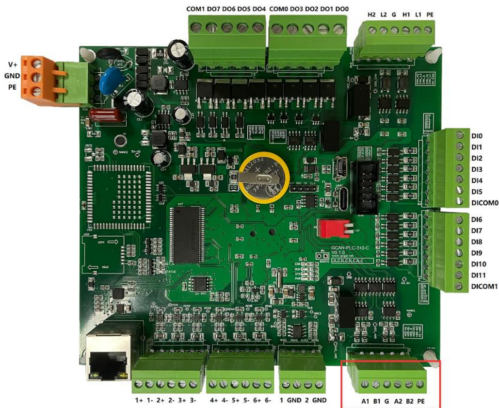
图 2.7 GCAN-PLC-310 的 RS485 接线图示
