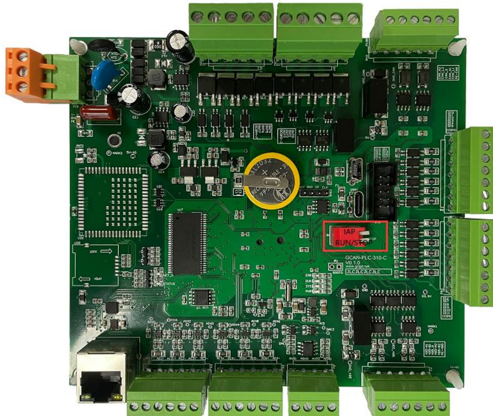
图 4.1 运行开关及复位键实物图
