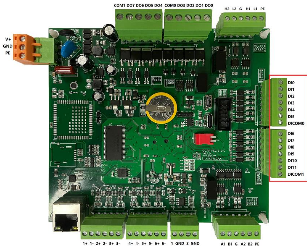
图 2.3 GCAN-PLC-310 的数字量输入 DI 接口样式
