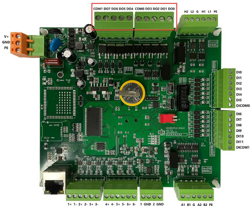
图 2.4 GCAN-PLC-310 的数字量输出 DO 接口样式
