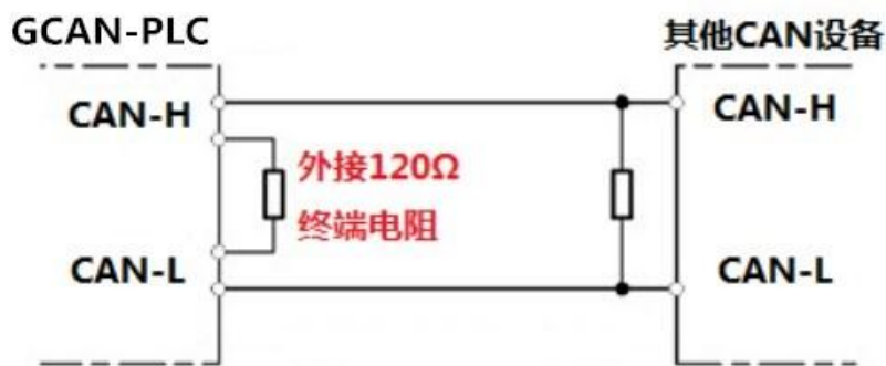
图 3.2 GCAN-PLC-310 模块与其他 CAN 节点设备连接
