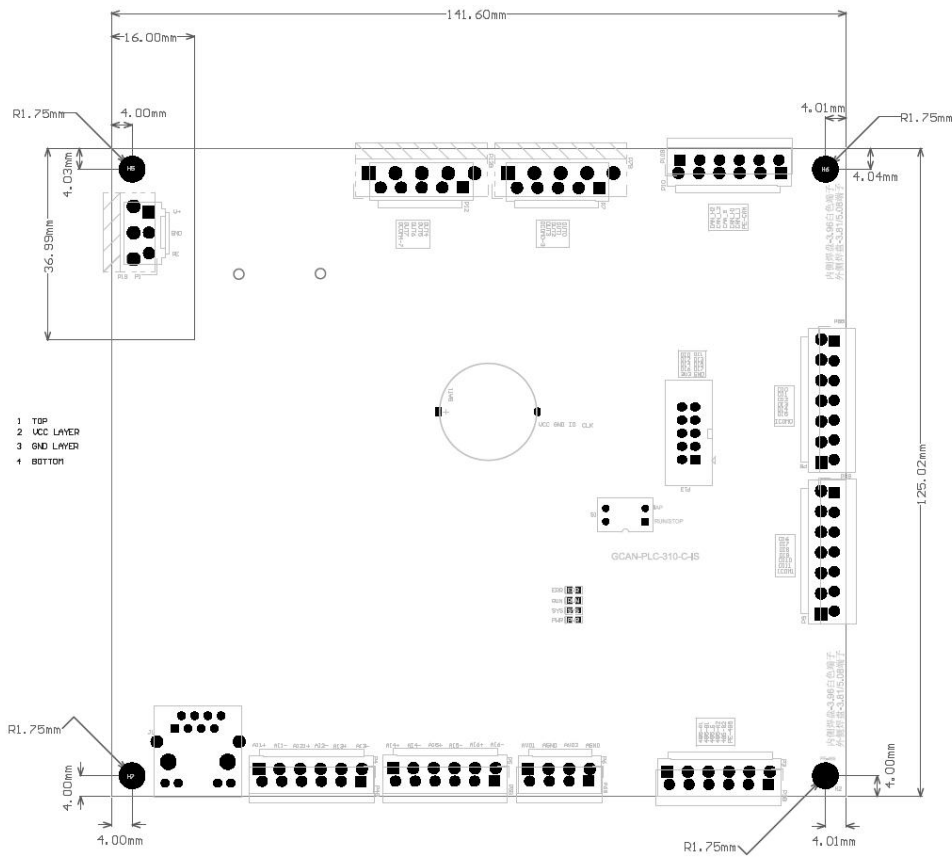
图 2.1 GCAN-PLC-310 外观尺寸图
