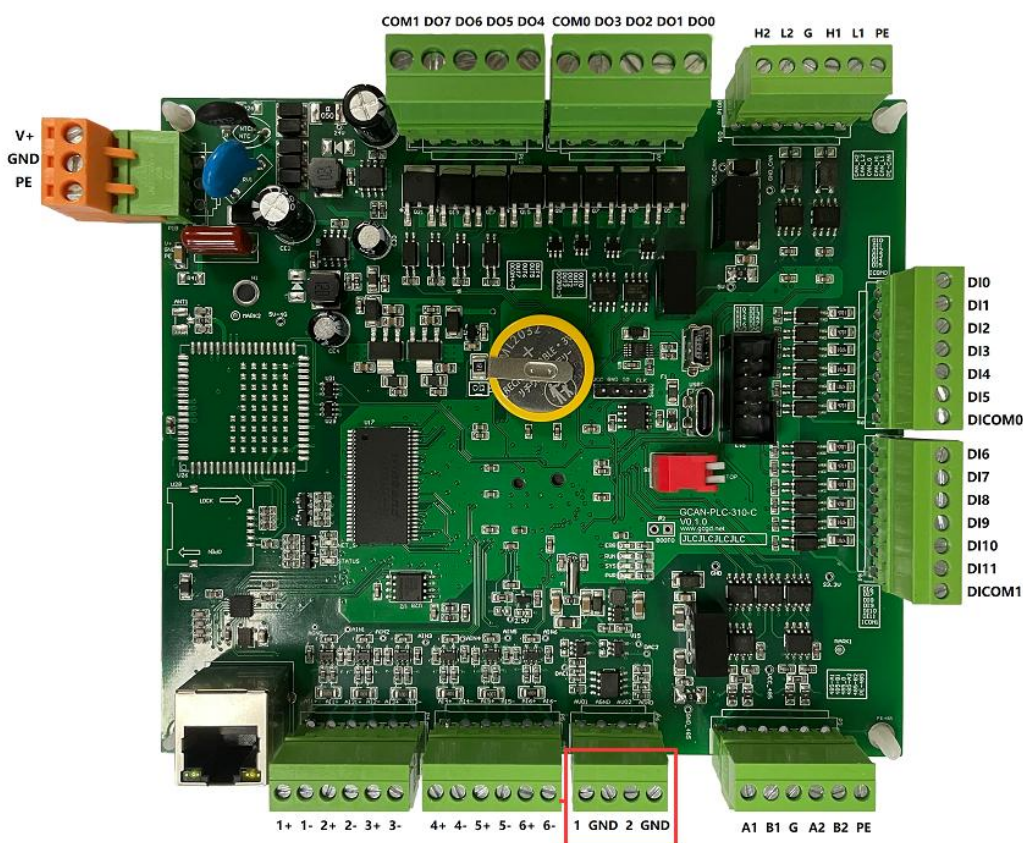
图 2.6 GCAN-PLC-310 的模拟量输出 AO 接口样式
