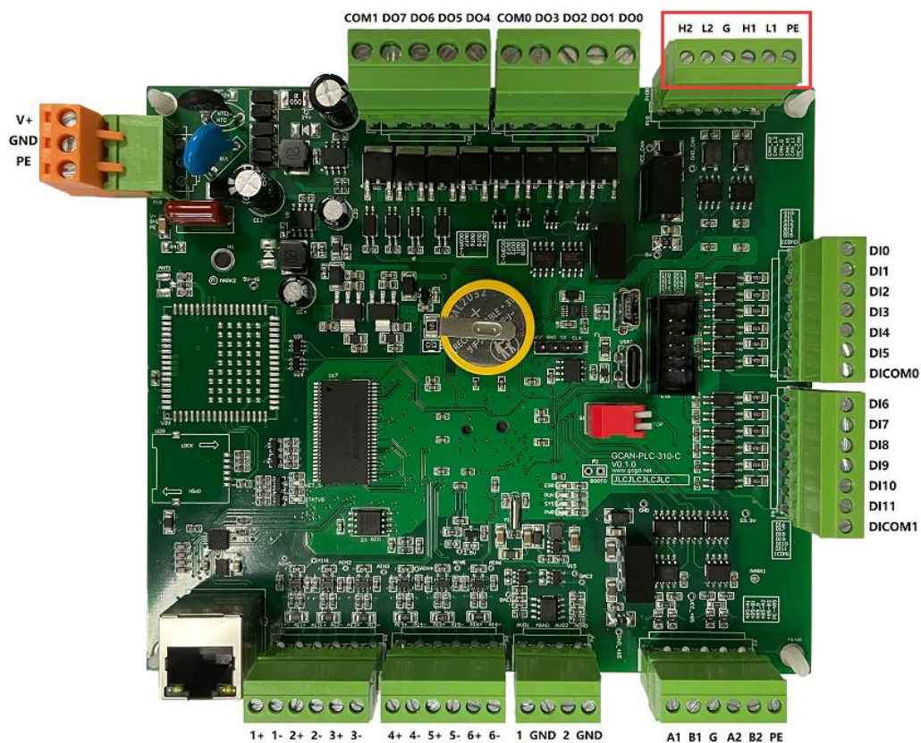
图 2.8 GCAN-PLC-310 的 CAN 总线接线图示
