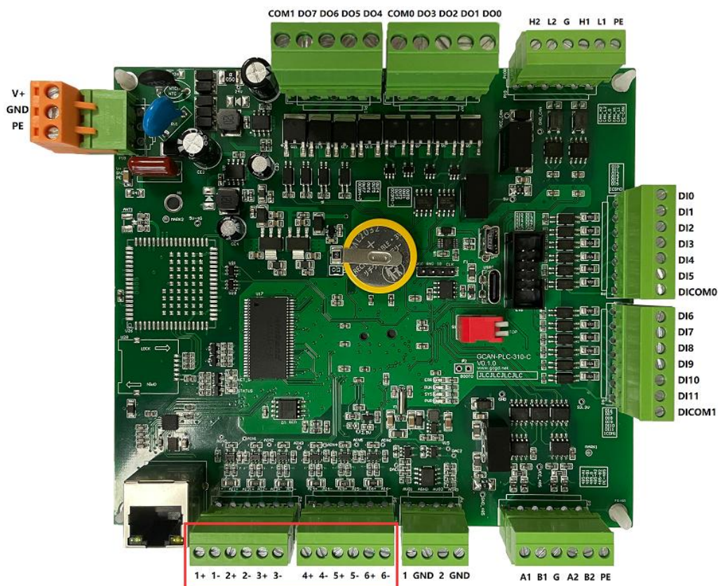
图 2.5 GCAN-PLC-310 的模拟量输入 AI 接口样式
