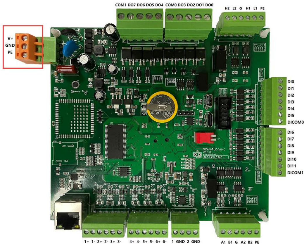
图 2.2 GCAN-PLC-310 的电源供电接口样式
