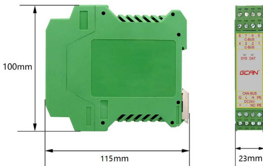
图 2.2 GCAN-204 模块外形尺寸
