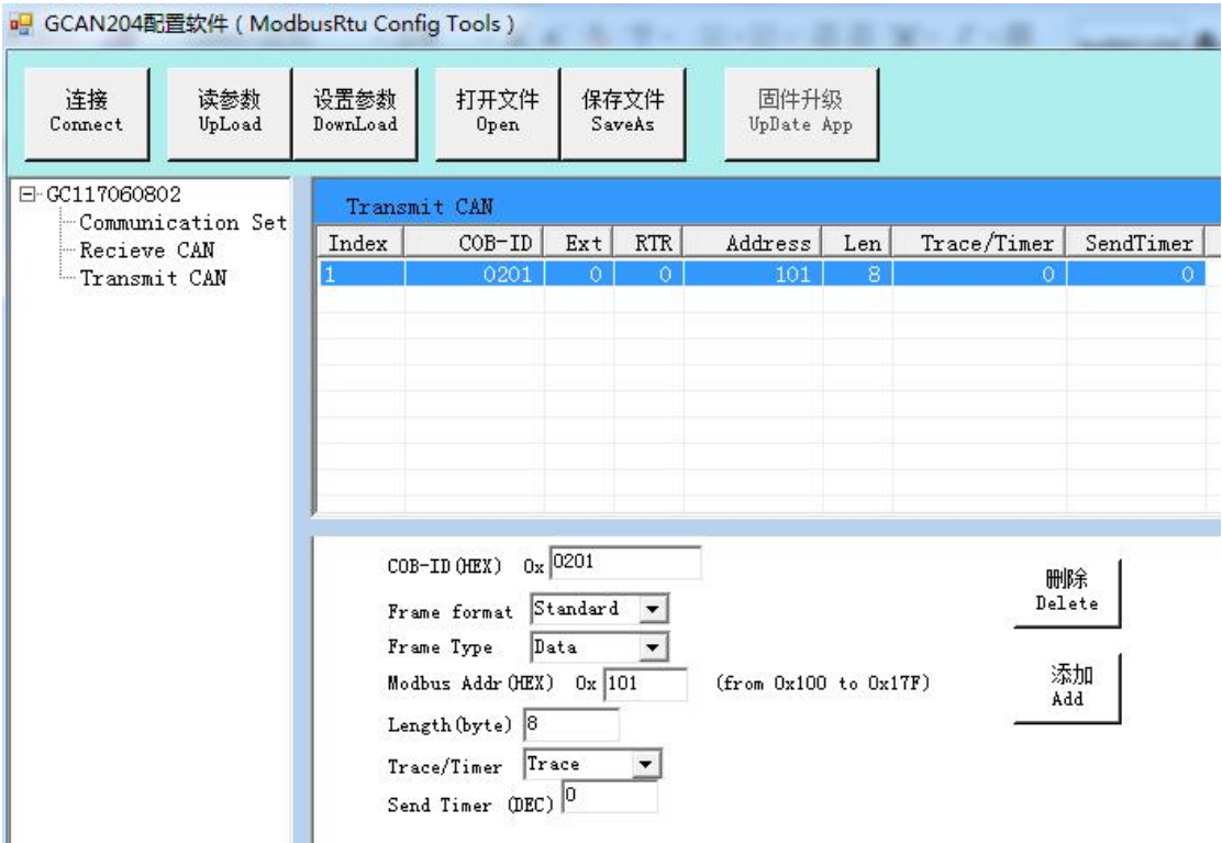
图 4.7 Transmit CAN 映射设置
