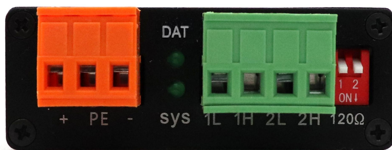
图 2.2 电源接口、CAN-bus 接口位置
