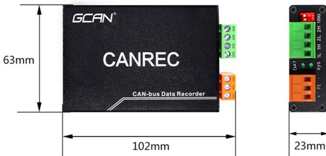
图 2.1 GCAN-402 模块外形尺寸
