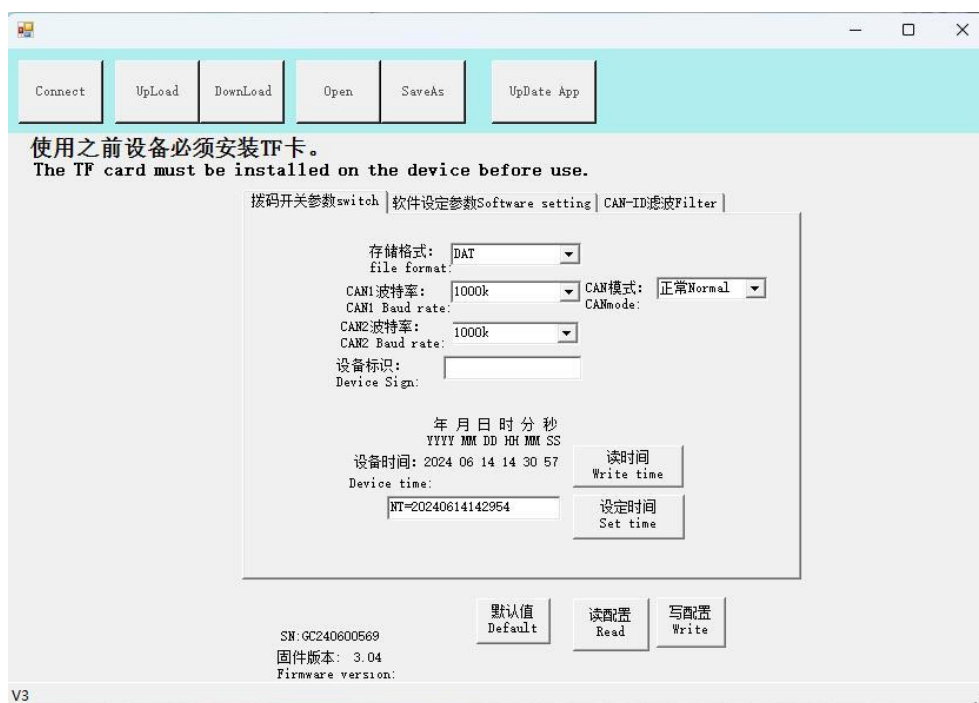
图3.3 拨码开关参数设置
