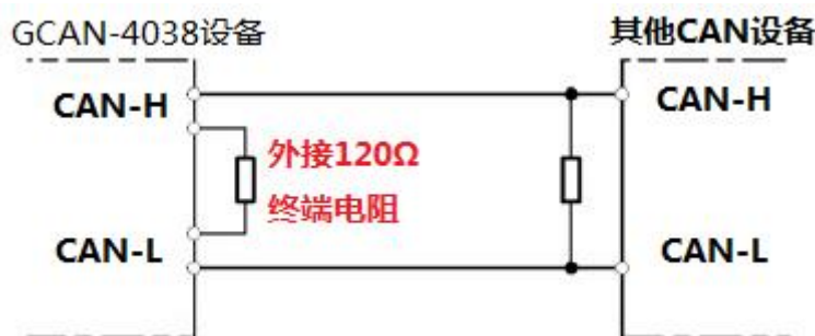
图 3.2 GCAN-4038 与其他 CAN 节点设备连接
