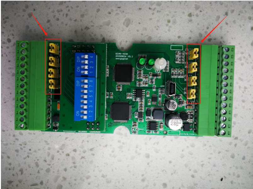
图 5.8 接上短接帽
