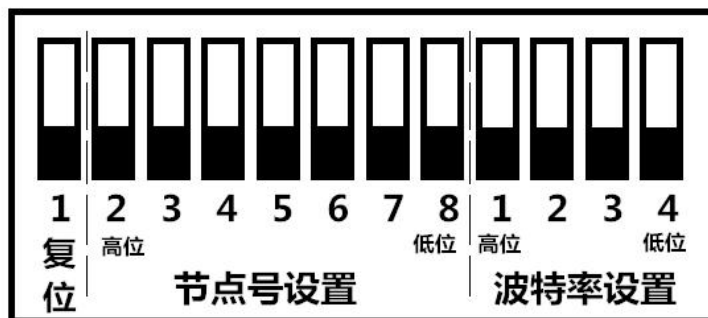
图 2.6 GCAN-4038 模块拨码开关
