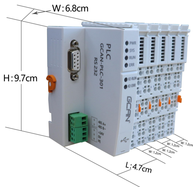
图 2.2 GCAN-PLC-302 外观尺寸图
