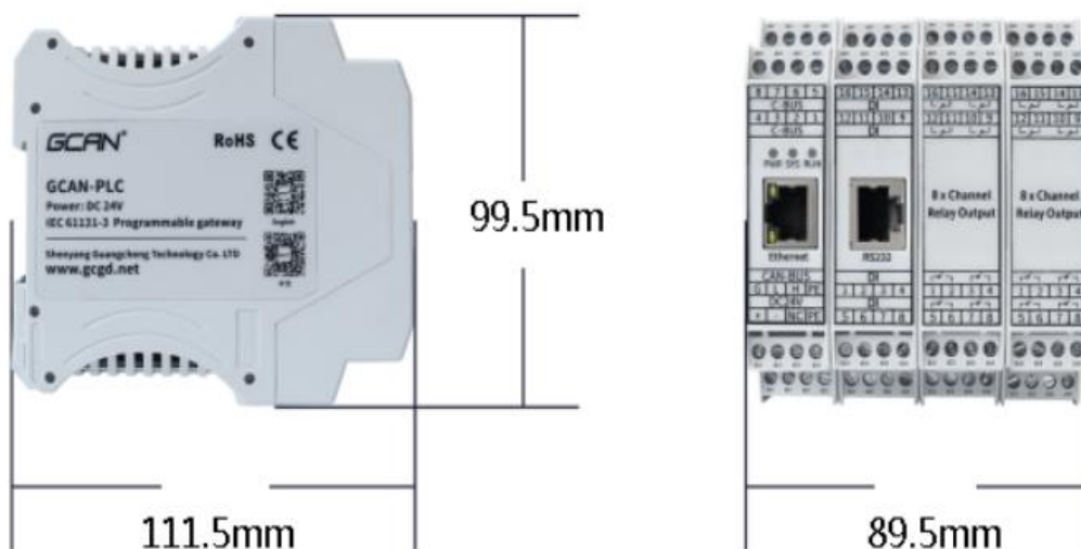
图 2.1 GCAN-GT-419 模块尺寸图
