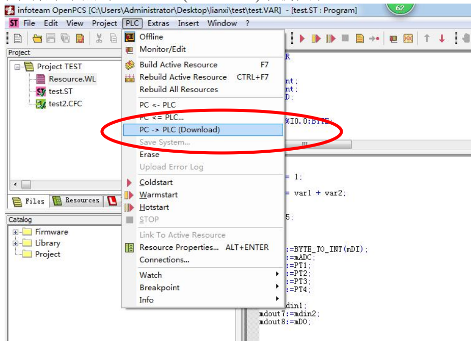
图 4.16 下载程序
