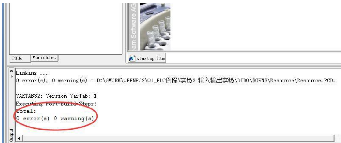
图 4.14 编译完成
