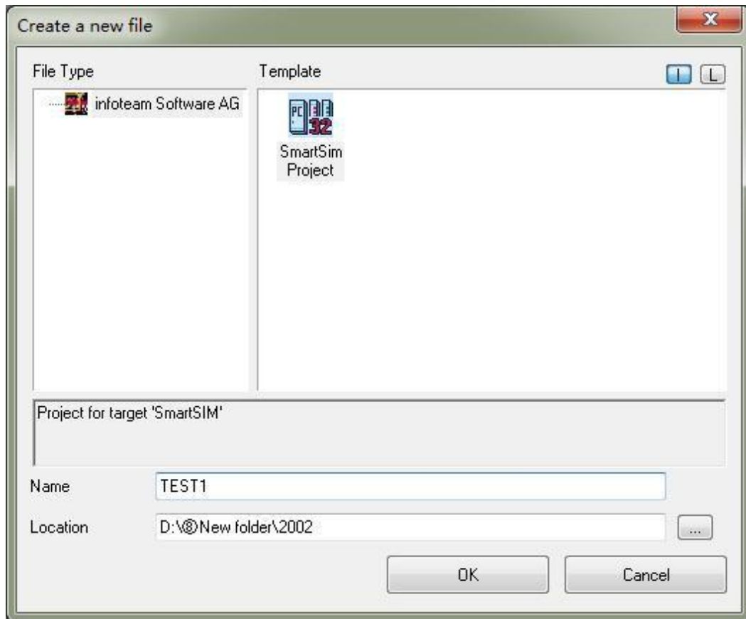
图 4.2 创建项目
