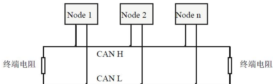
图 3.1 CAN-bus 网络的拓扑结构
