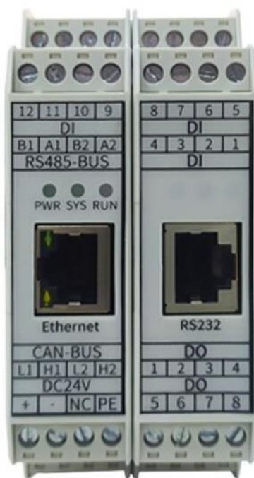
图 2.3 GCAN-GT-413 模块接线端子排
