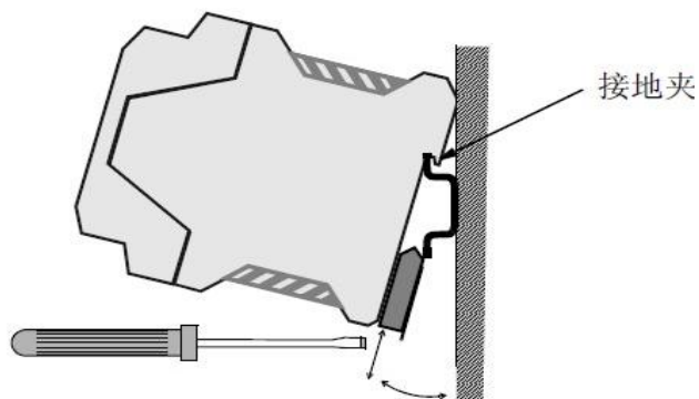
图 2.2 GCAN-GT-413 模块安装
