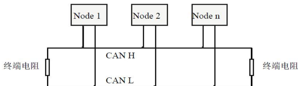
图 3.1 CAN-bus 网络的拓扑结构
