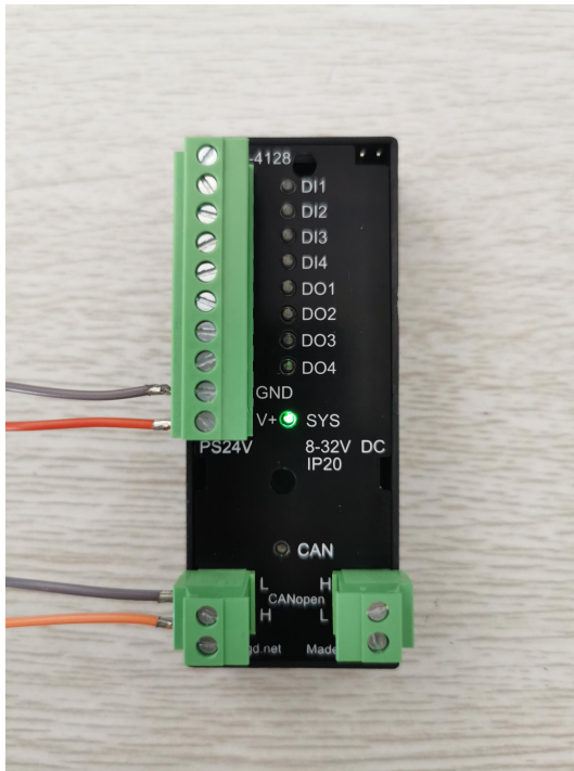
图 3.1 GCAN-4128 SYS 指示灯状态
