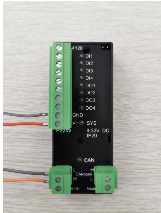
图 3.1 GCAN-4128 SYS 指示灯状态
