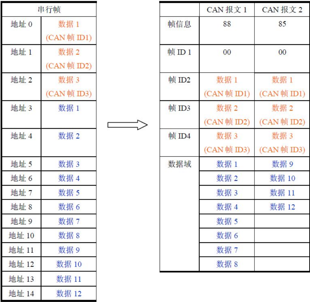
图 5.8 串行帧转 CAN 报文示例（透明带标识转换）
