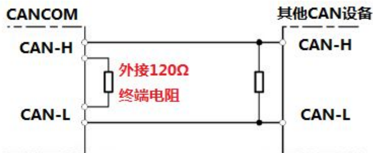
图 3.2 GCAN-207 与其他 CAN 节点设备连接
