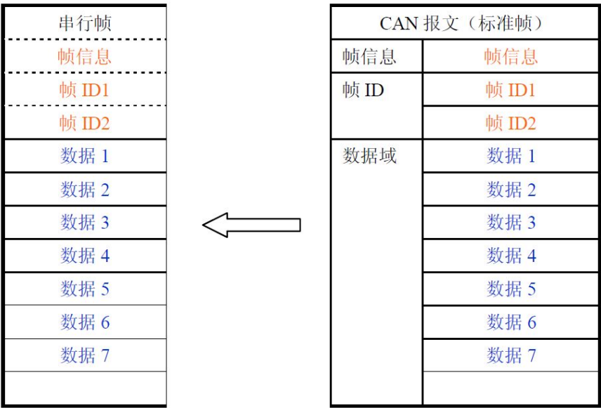
图 5.2 CAN 报文转换成串行帧（透明转换）
