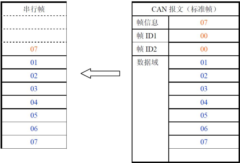
图 5.4 CAN 报文转串行帧示例（透明转换）
