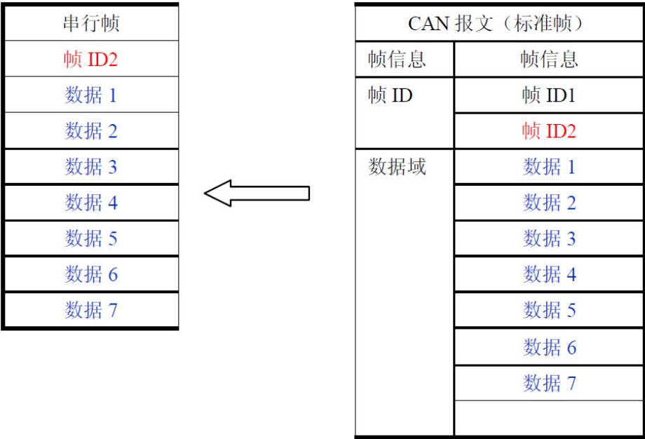
图 5.7 CAN 报文转串行帧（透明带标识转换）
