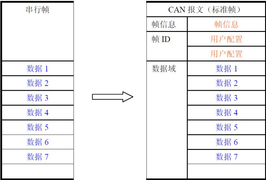
图 5.1 串行帧转换成 CAN 报文（透明转换）
