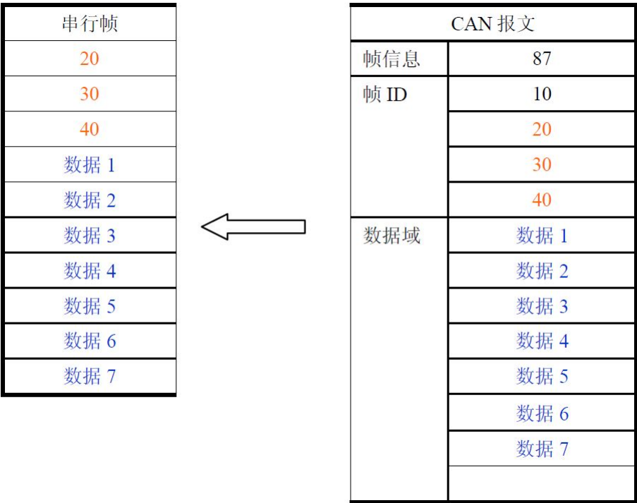
图 5.9 CAN 报文转串行帧示例（透明带标识转换）
