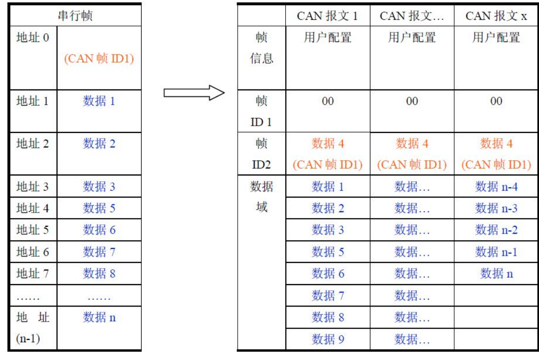
图 5.6 串行帧转 CAN 报文（透明带标识转换）
