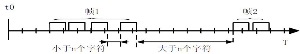
图 5.5 串行帧时间格式（透明带标识转换）
