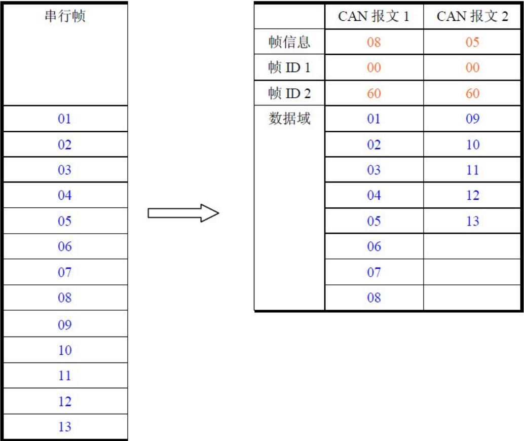
图 5.3 串行帧转 CAN 报文示例（透明转换）
