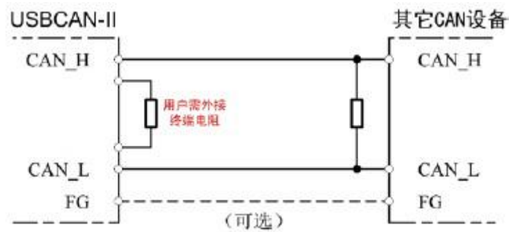
图 3.2 USBCAN-II FD 与其他 CAN 节点设备连接
