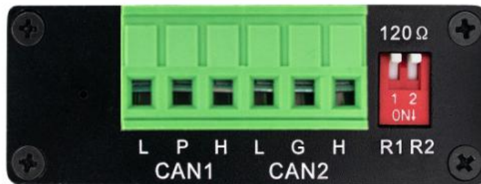
图 2.3 CAN (FD) -bus 接口位置
