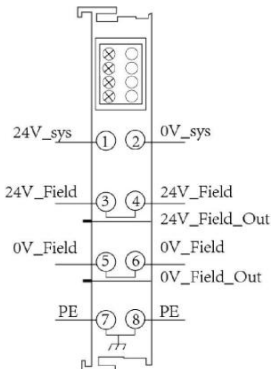
图 2.4 GCAN-8100 模块接线端子排
