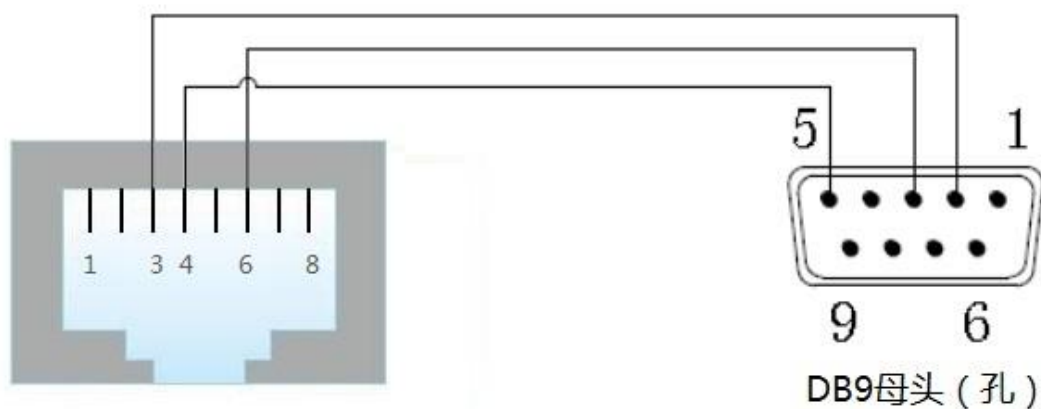
图 2.5 GCAN-PLC 的 RS-232 接口样式
