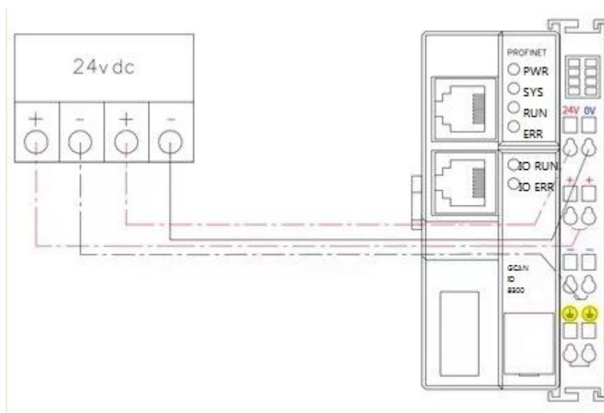
图 2.1 GCAN-IO-8300 Profinet 总线耦合器外观图
