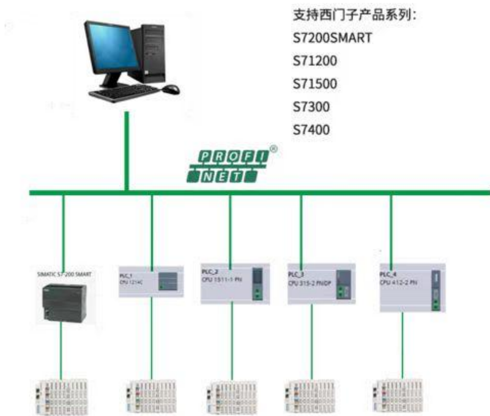
图 3.1 GCAN-IO-8300 Profinet 总线耦合器与多种 Profinet 控制器接入总线
