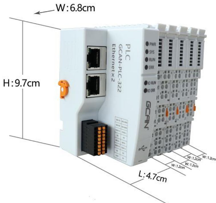
图 2.2 GCAN-PLC-322 外观尺寸图
