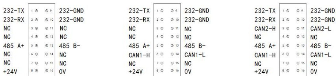
图 2.7 GCAN-PLC-320/321/322 的通信与供电接口样式
