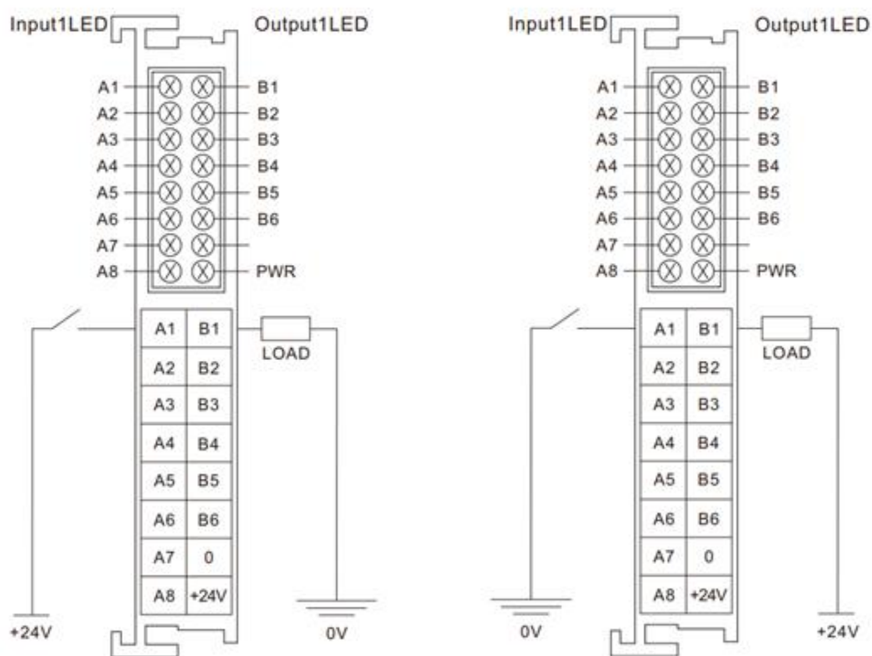
图 2.8 PNP 型接线端子排
