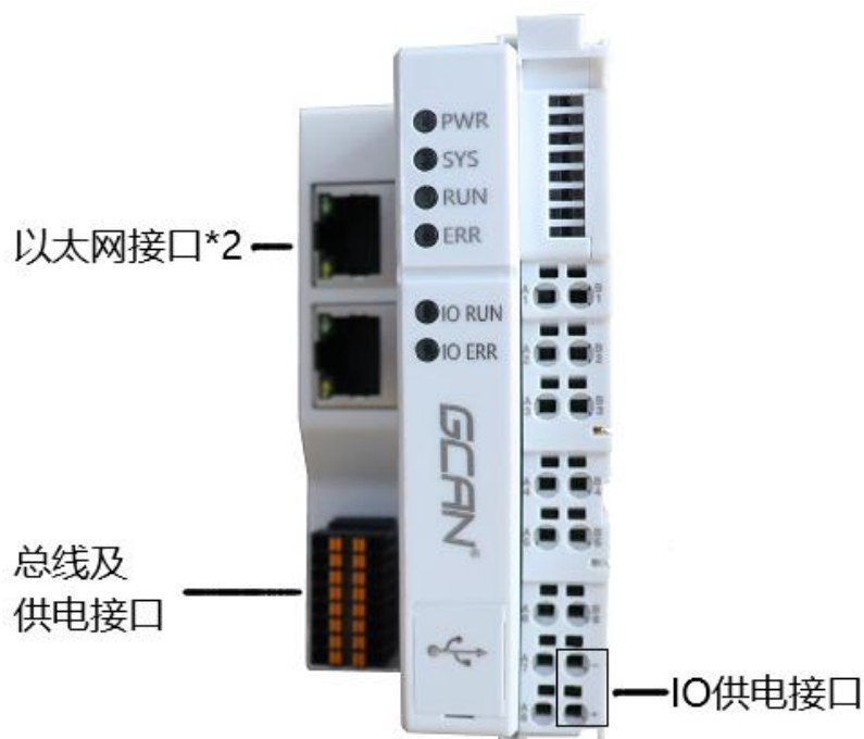
图 2.1 GCAN-PLC-322 外观接口图
