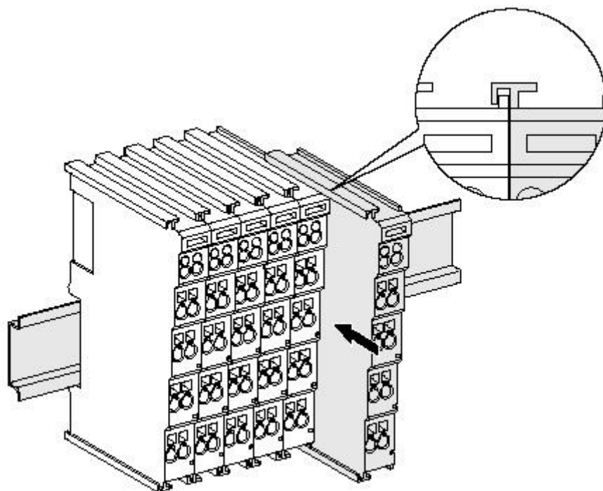
图 2.3 GCAN-PLC-IO 安装
