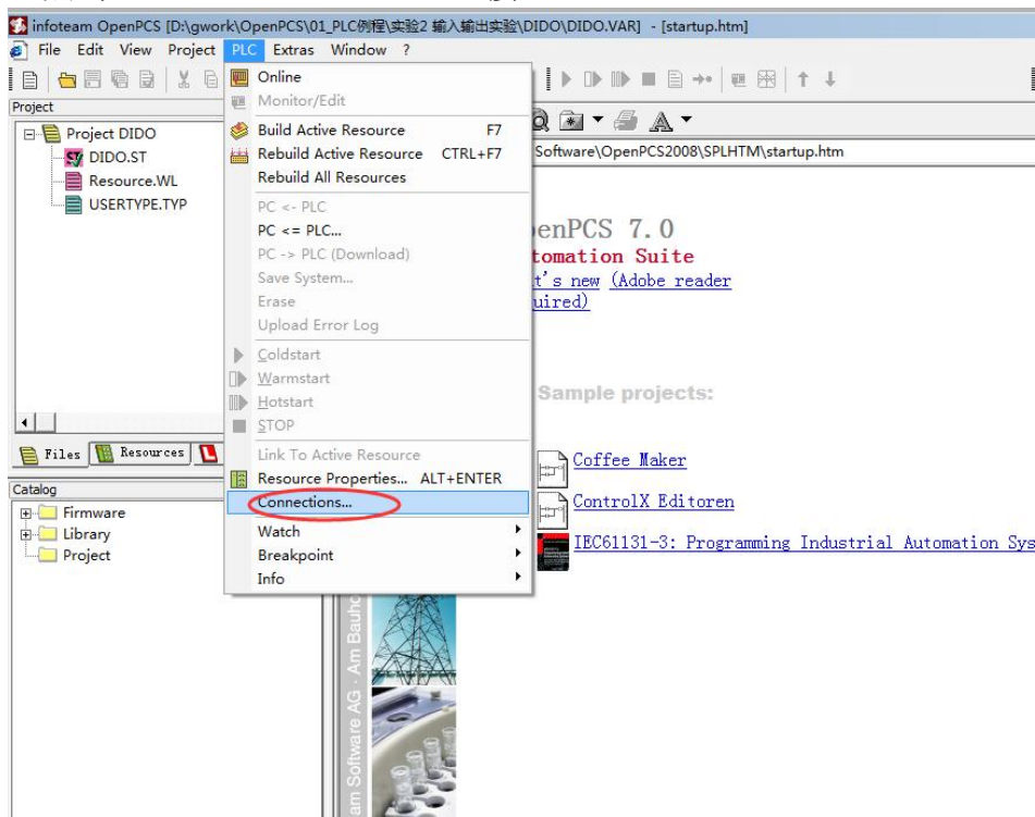
图 6.4 调试连接
