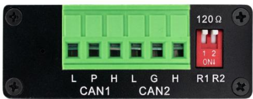
图 2.3 CAN（FD）-bus 接口位置
