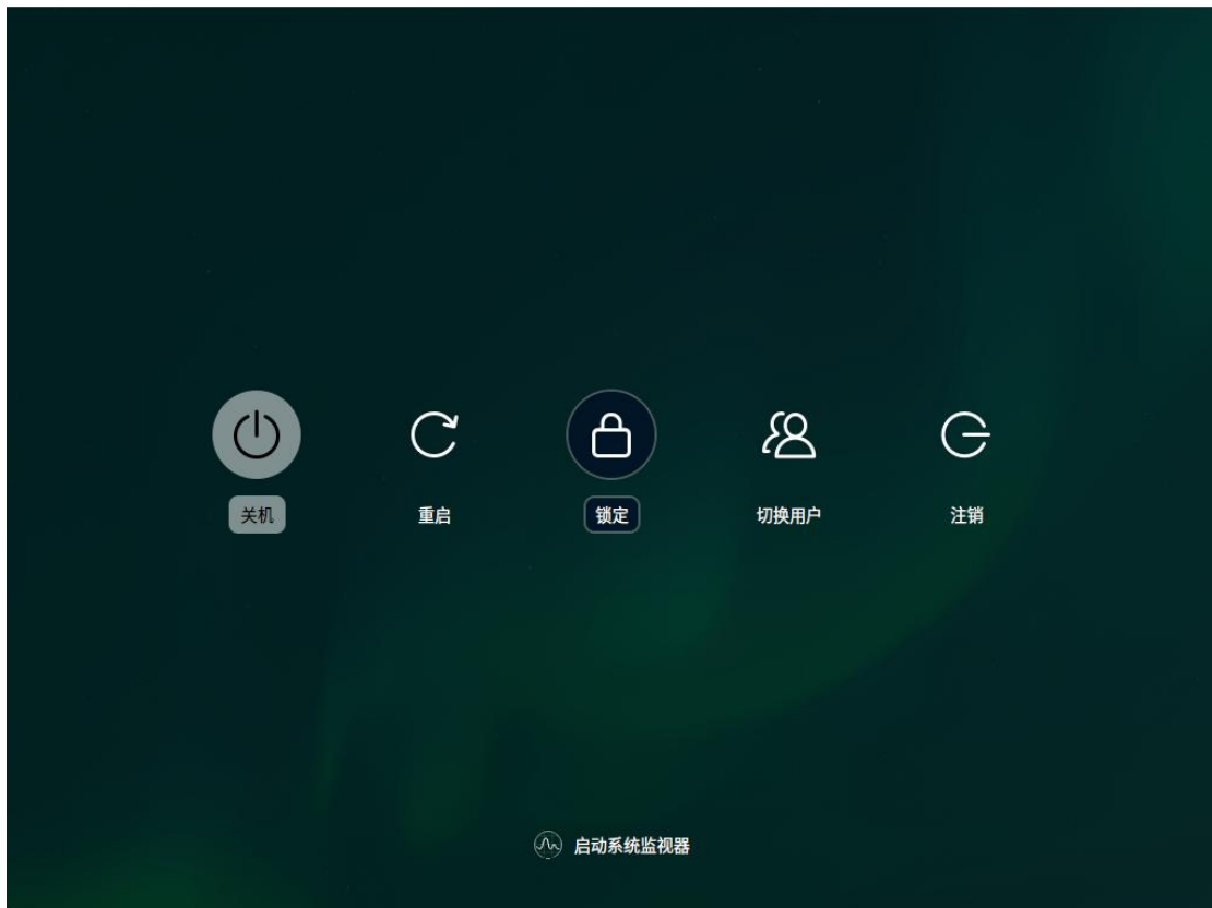
图 1.4.1 关机
