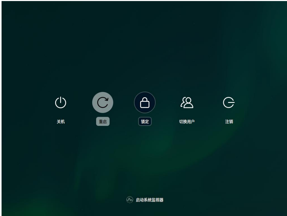
图 1.4.2 重启
