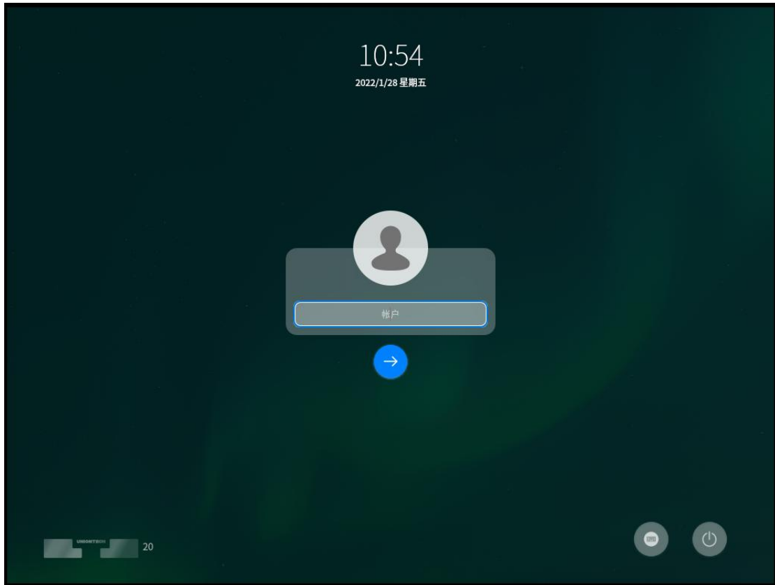
图 1.1.2 登录界面
