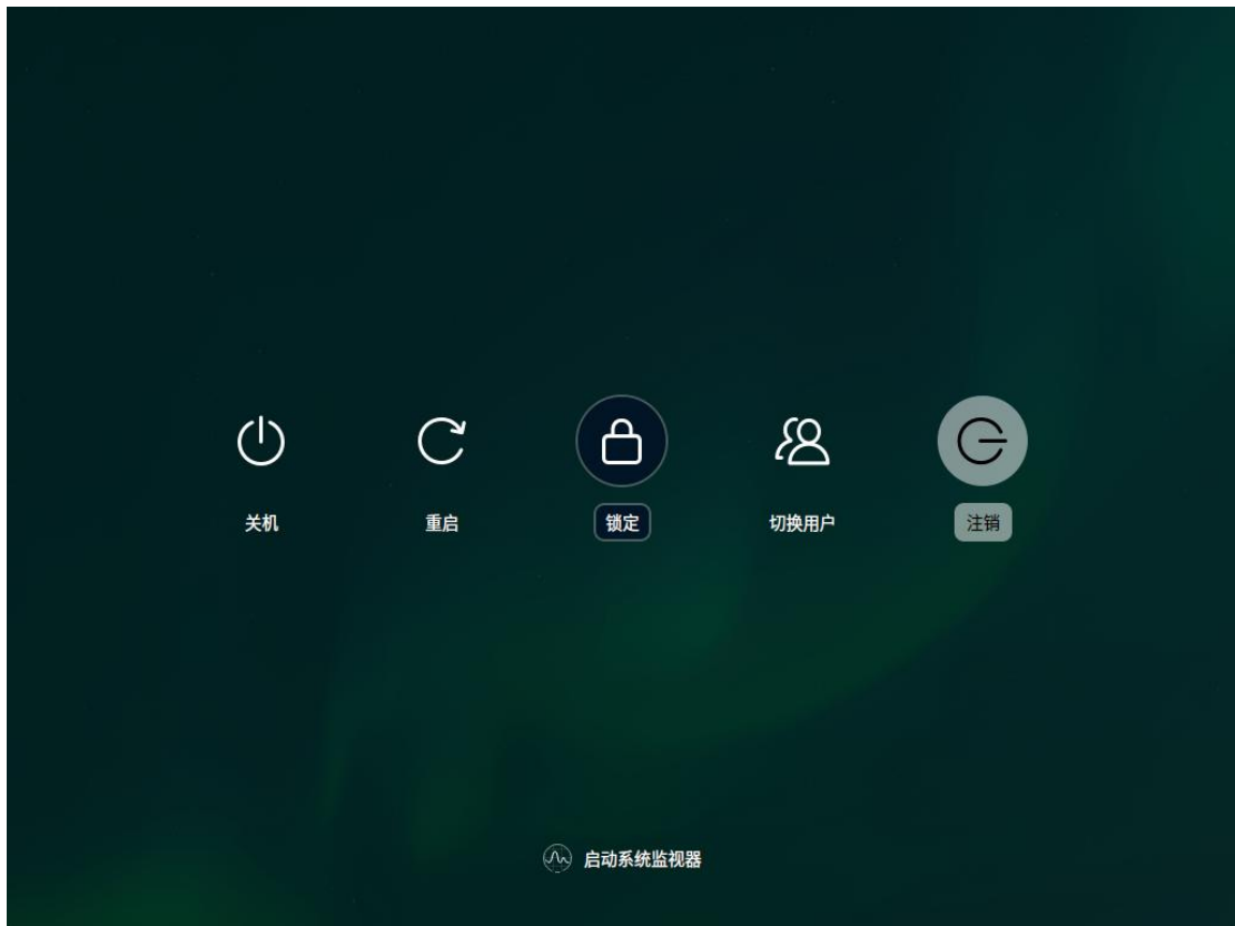
图 1.3.1 注销
