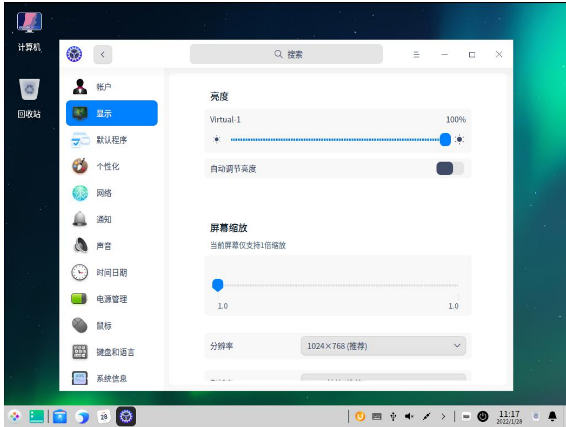
图 1.6.2 设置分辨率
