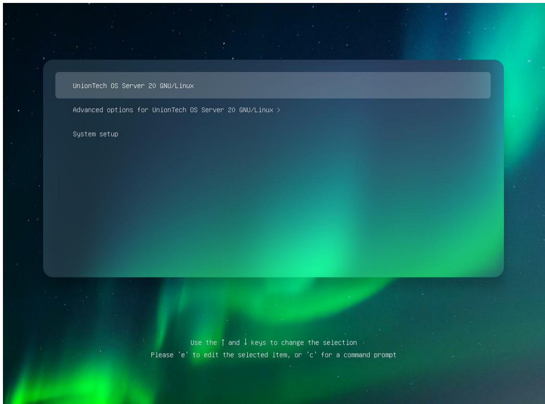
图 1.1.1 Grub 界面
