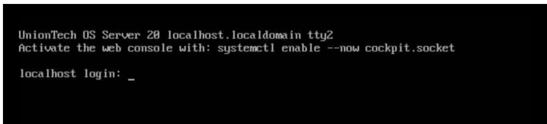
图 1.5.1 字符界面
