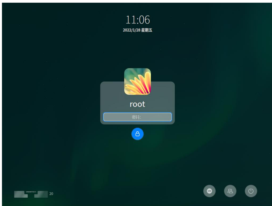
图 1.5.2 图形界面
